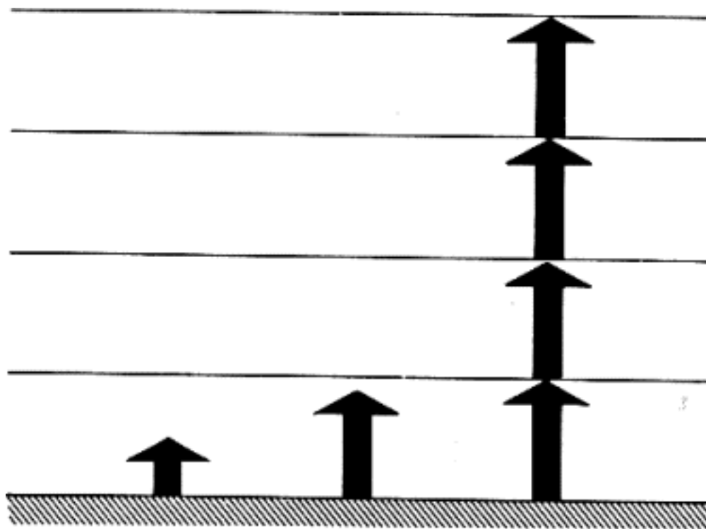
Рис. 5.1. Эффект лестницы
