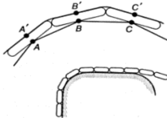
Рис. 1.9. Модель щупальца
