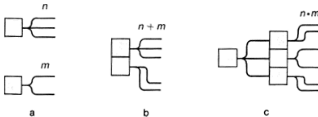
Рис. 9.6. Действия над целыми числами
