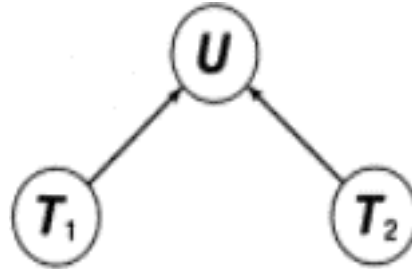
Рис. 3.3. Ассоциация представлений
