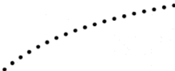
Рис. 3.4. точки образуют линию
