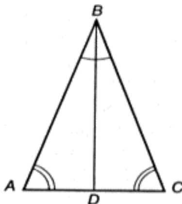
Рис. 10.1. Равнобедренный треугольник
