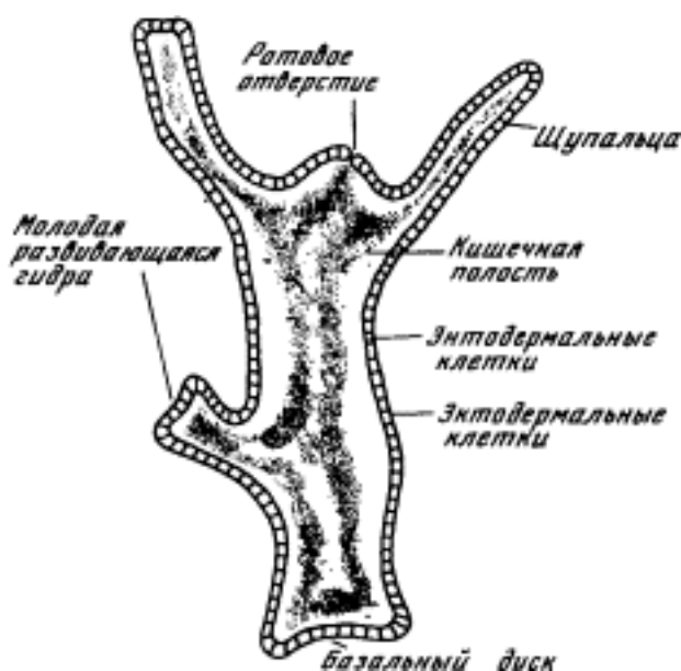
Рис. 1.8. Строение гидры
