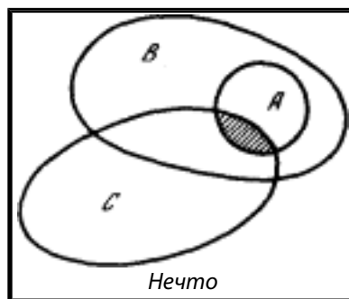
Рис. 6.4. Схема умозаключения disamis
