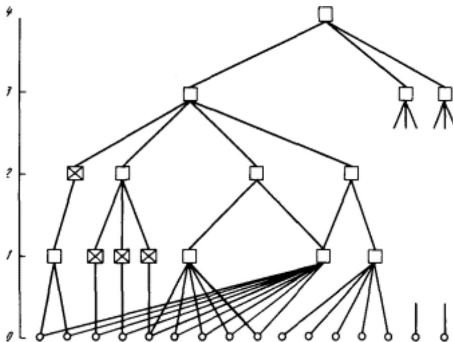
Рис. 2.2. Иерархия классификаторов
