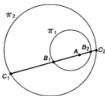
Рис. 10.6. К доказательству теоремы T_1
