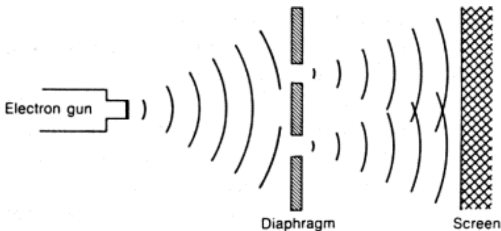
Рис. 13.1. Дифракция электронов
