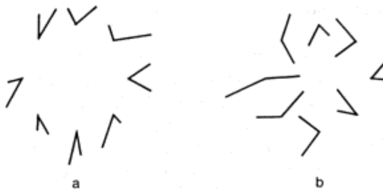
Рис. 3.5. Маскировка круга, образуемого вершинами углов
