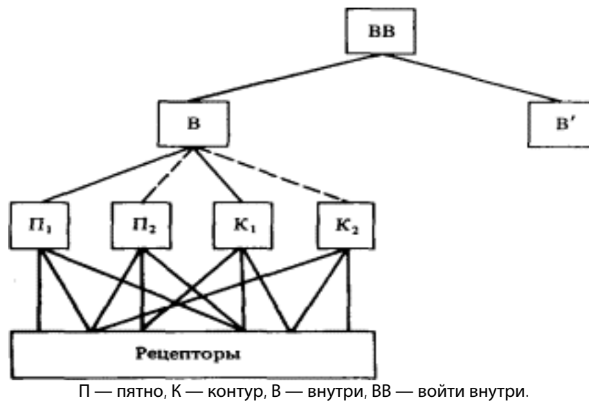
Рис. 7.4. Иерархия классификаторов
