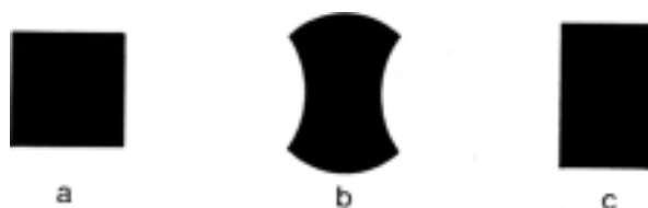
Рис. 3.6. Иллюзия сближения диагоналей
