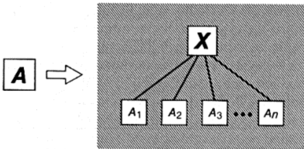
Рис. 3.1. Метасистемный переход
