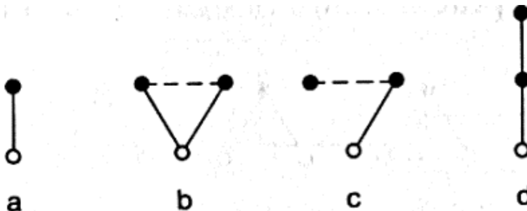
Рис. 2.8. Редупликация эффекторов
