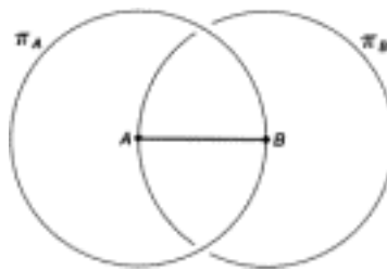
Рис. 10.4. «Перескакивающие» окружности
