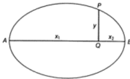
Рис. 11.3. Ордината и абсциссы эллипса
