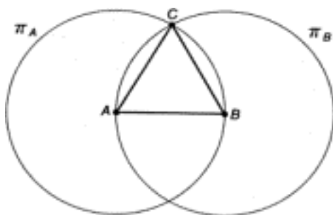
Рис. 10.3. Построение равностороннего треугольника
